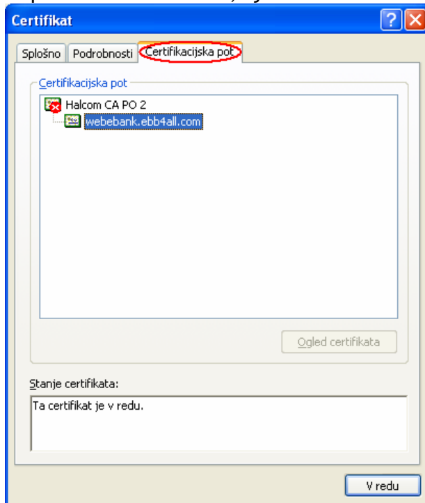
Slika 6: Izbira certifikata
