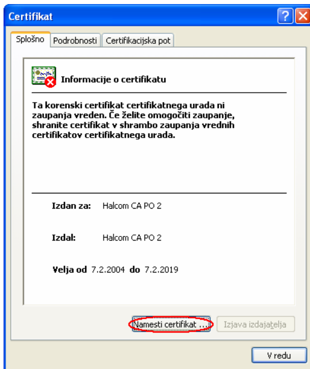
Slika 8: Namestitev certifikata
