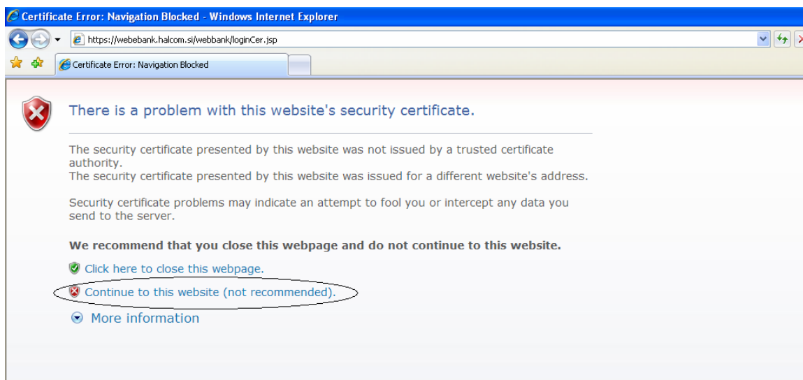
Slika 1: Opozorilo
