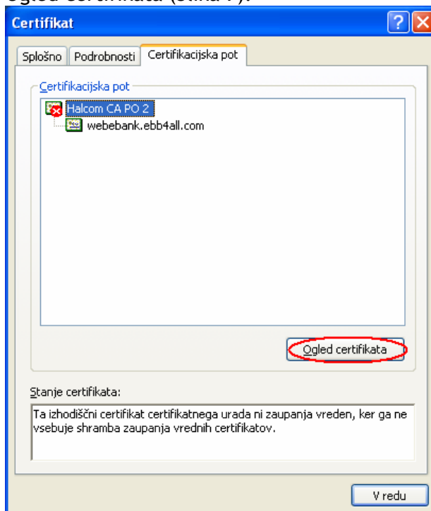
Slika 7: Ogled certifikata
