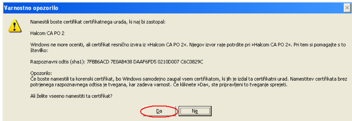
Slika 10: Varnostno opozorilo
