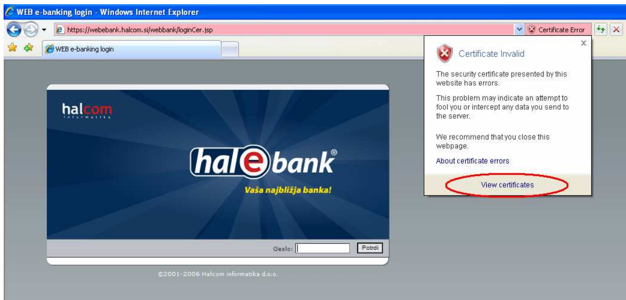
Slika 5: Ogled certifikatov
